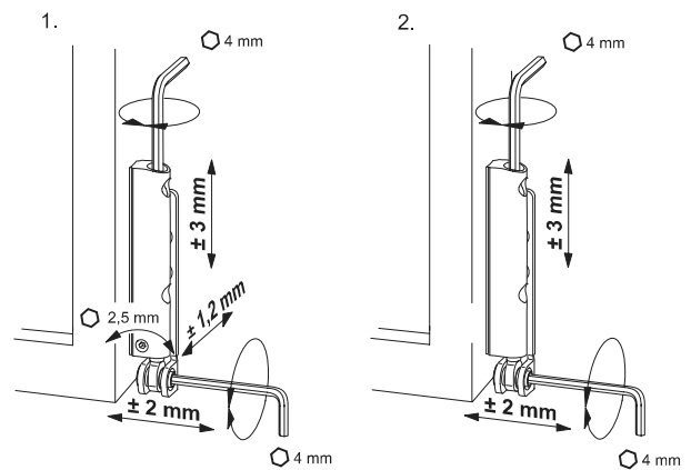
1. С регулировкой прижима 2. Без регулировки прижима
