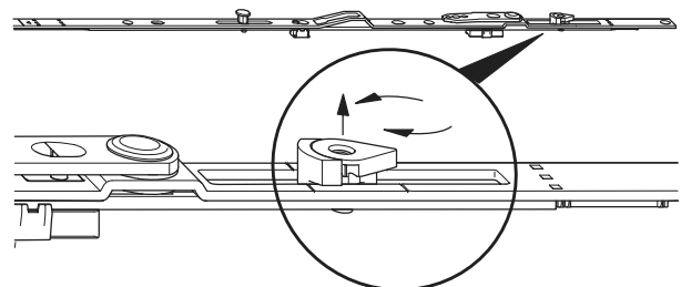
Доводчик закрывания створки в положении наклона
